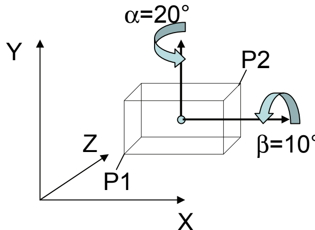
Abbildung 1: Rotation in 3D (siehe Aufgabe 8-2)
